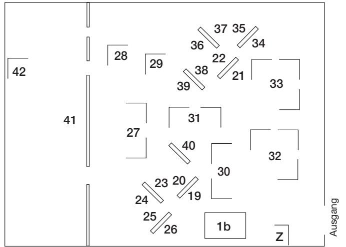
Gebäude A5 // Galerien
